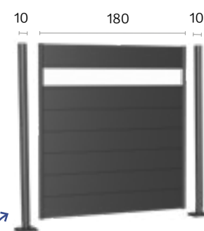
Brise-vue composé de : 1 panneau droit avec lames et 2 poteaux
