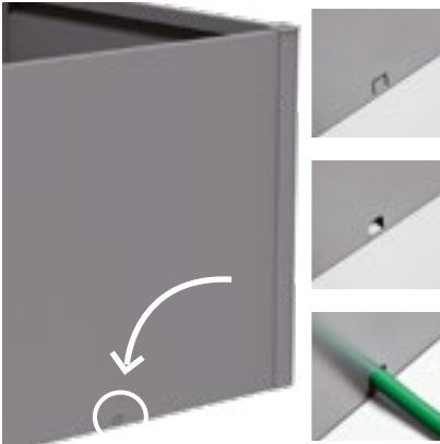
02 Préparation pour tuyau d'irrigation
