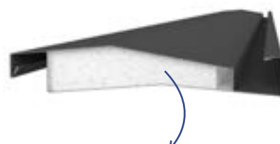
Structure des lamelles Construction en sandwich avec âme en Peripor
