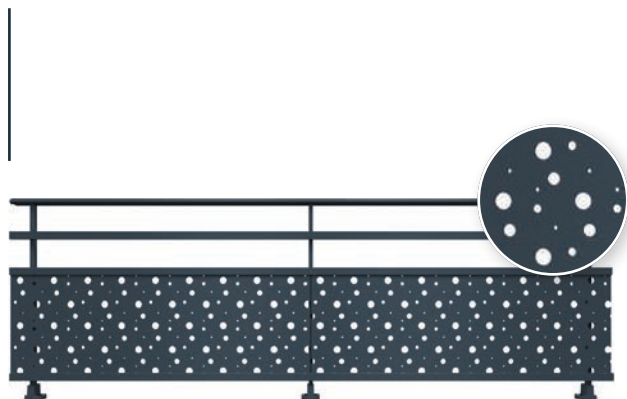
Style : lisse intermédiaire horizontale 25 x 15 mm, tôle perforée motif bulles de savon Coloris : gris anthracite RAL 7016 FT
