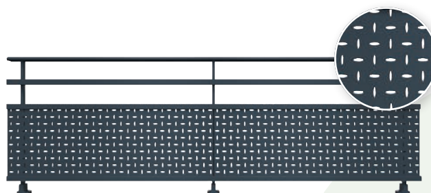
Style : lisse intermédiaire horizontale 25 x 15 mm, tôle perforée motif oblong Coloris : gris anthracite RAL 7016 FT
