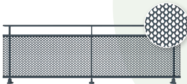
Style : tôle perforée motif Écaille Coloris : gris anthracite RAL 7016 FT
