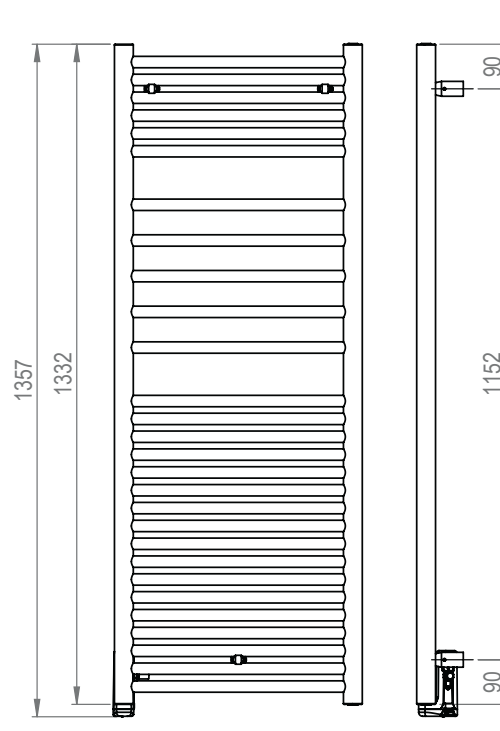
Saillie au mur : 94 mm
