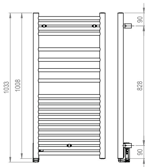
Vue de face 500 W :
