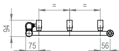
Saillie au mur : 94 mm
