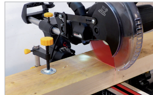
Butée de profondeur de coupe pour le rainurage Depth cutting gauge for grooving
