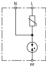
Schéma de principe du circuit DG TT 2P 5 275 NL
