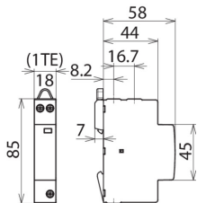
Dimensions DG TT 2P 5 275
