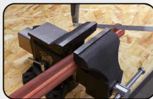
Mâchoires inférieures pour serrage de tubes Lower jaws for tube clamping
