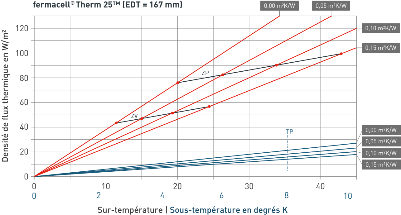
Diagramme de caractéristiques pour une chape intégrant le plancher chauffant fermacell® Therm 25™ (EDT = 167 mm)
