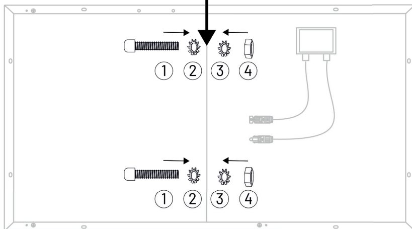
Vis de renfort des panneaux x2 (par panneau)
