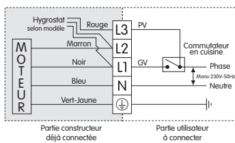
Schéma de câblage avec interrupteur
