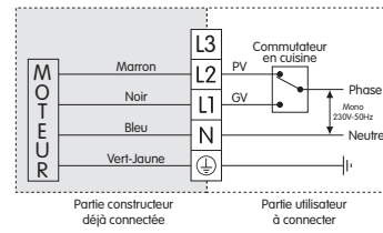
Schéma de câblage avec inverseur
