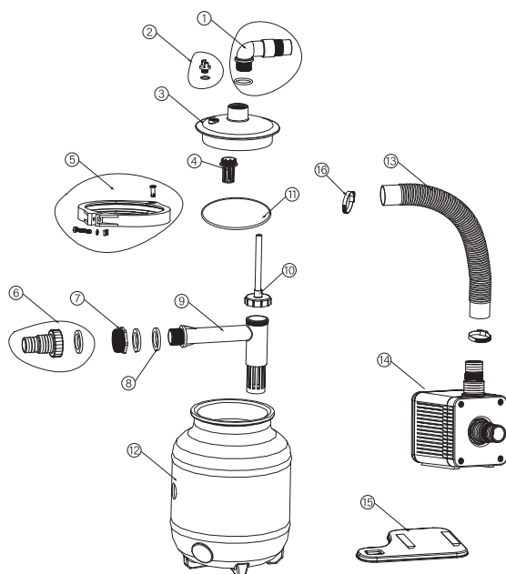
PIÈCES DE RECHANGE FIGURE E1/L1 SPARE PARTS ILLUSTRATION E1/L1 ERSATZTEILE ABBILDUNG E1/L1
