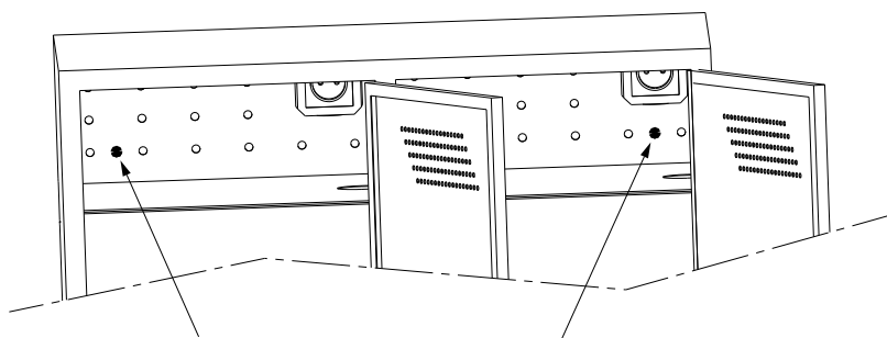
Trous de fixation mural, antibasculement
